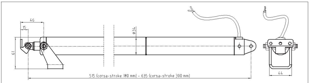
Actuators dimensions
